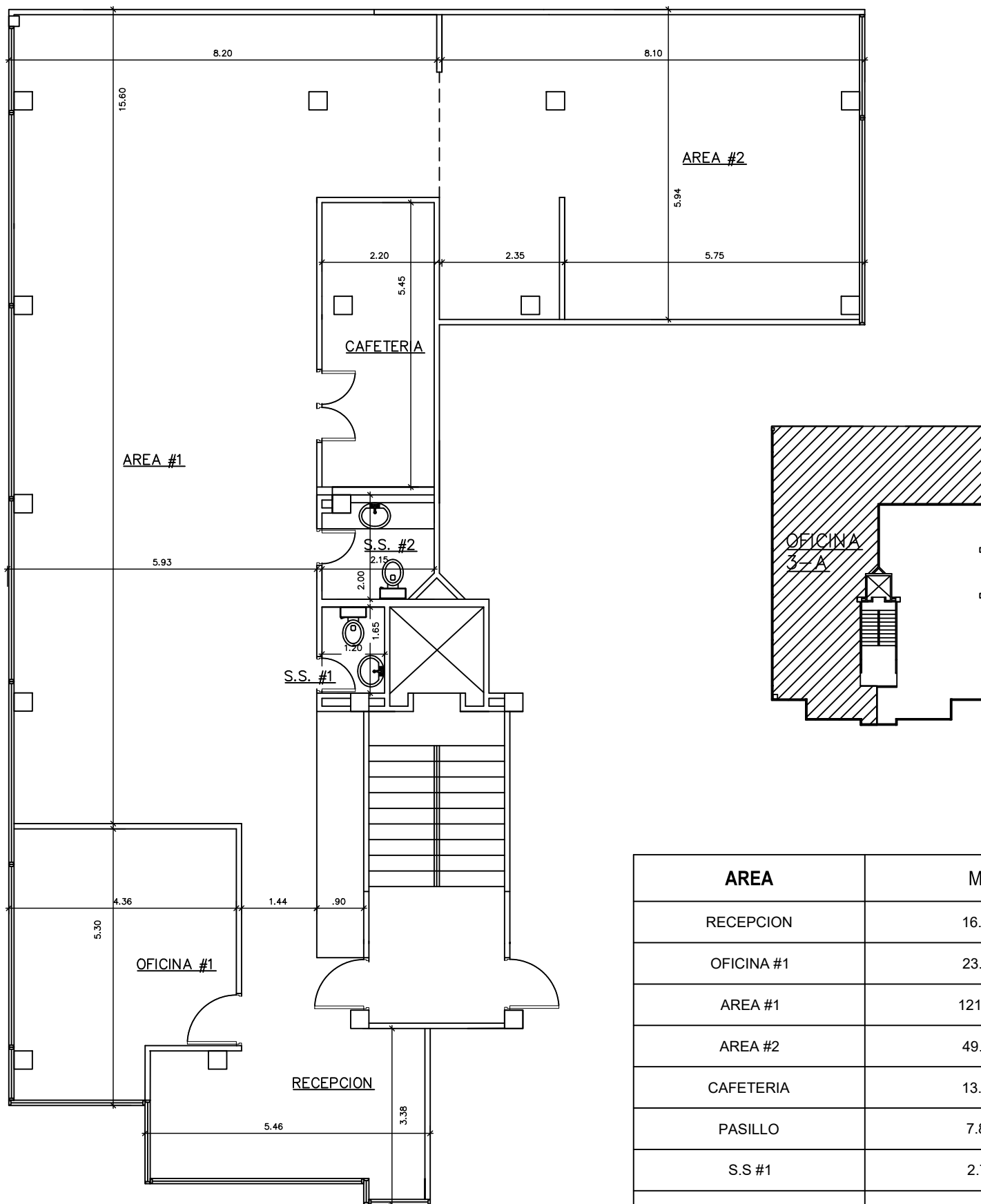
OFICINA 3-A ESC. 1:100
